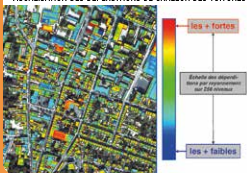
VISUALISATION DES DÉPERDITIONS DE CHALEUR DES TOITURES
